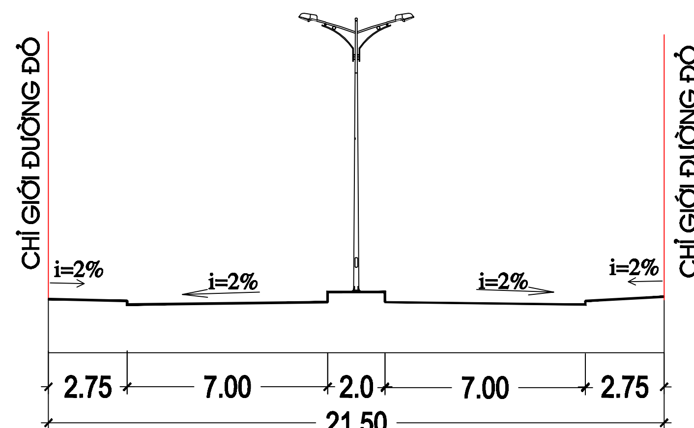
MẶT CẮT ĐƯỜNG TRƯỜNG CHINH (ĐOẠN TỪ ĐƯỜNG LÊ HỒNG PHONG ĐẾN ĐƯỜNG PHAN ĐÌNH PHÙNG)
