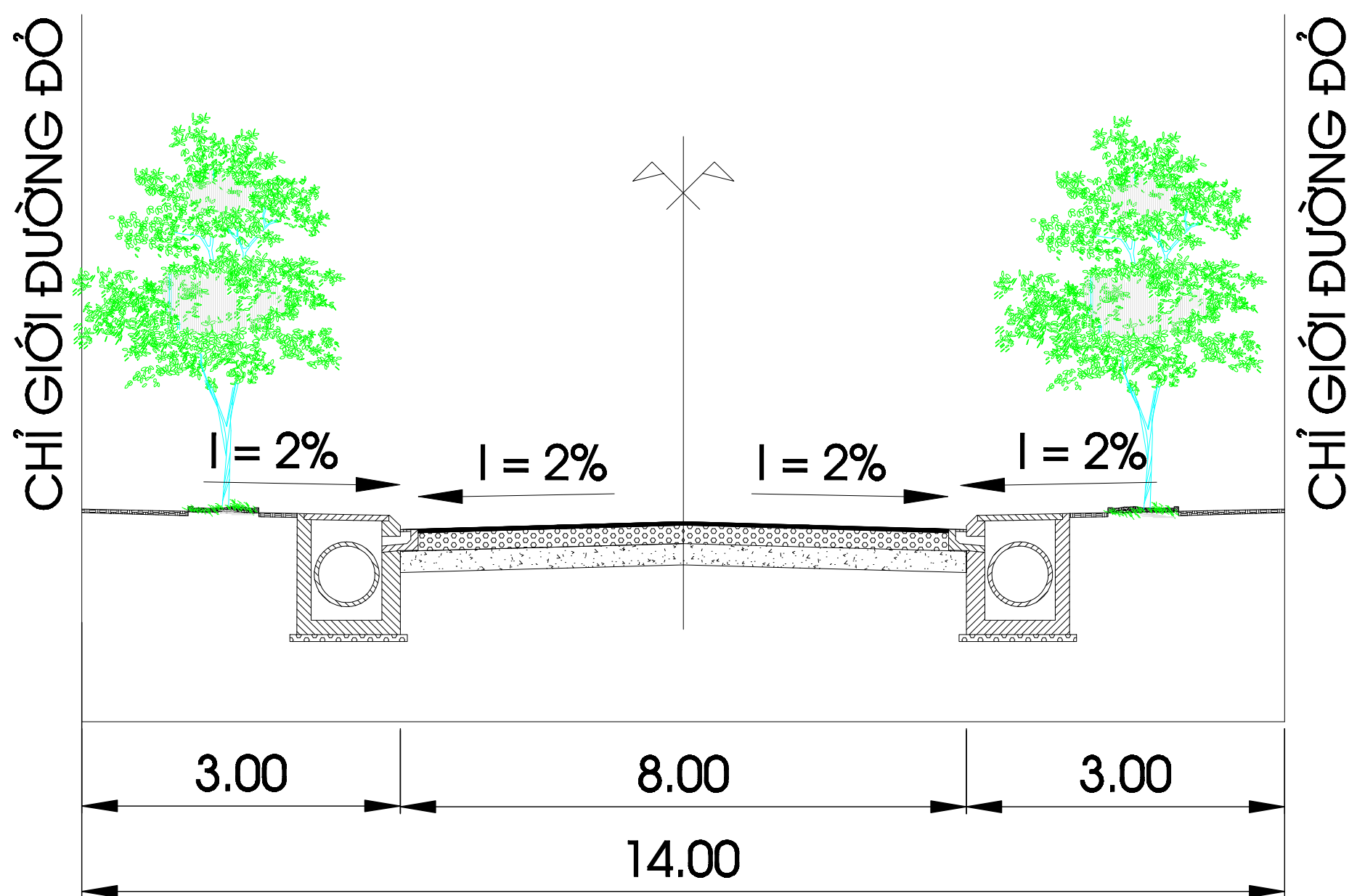
MẶT CẮT 9-9
